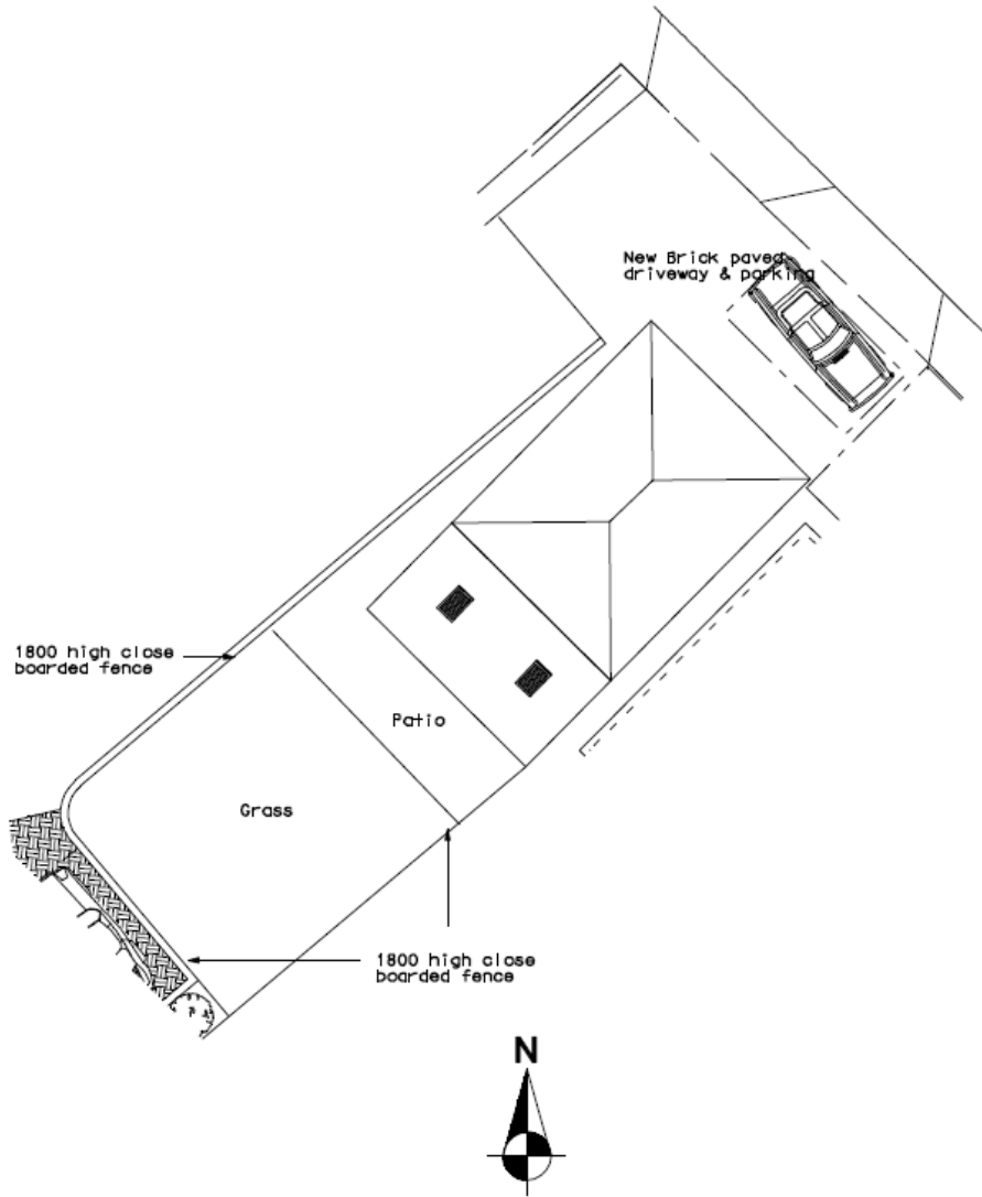
SITE PLAN (1:200)
